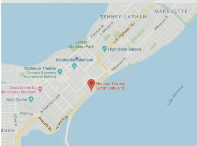
MAP
